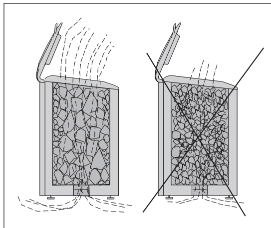
Figure 4. Piling of the sauna stones Abbildung 4. Aufsichtung der Saunafensteine
