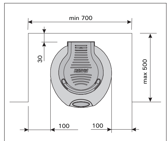
Figure 8. Installation of the heater in a recess Abbildung 8. Montage des Saunaofens in einer Wandnische
